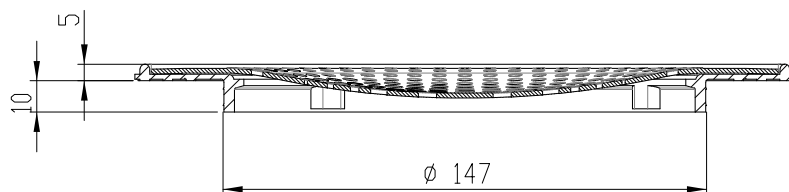
SECTION A-A SCALE 1 : 2
